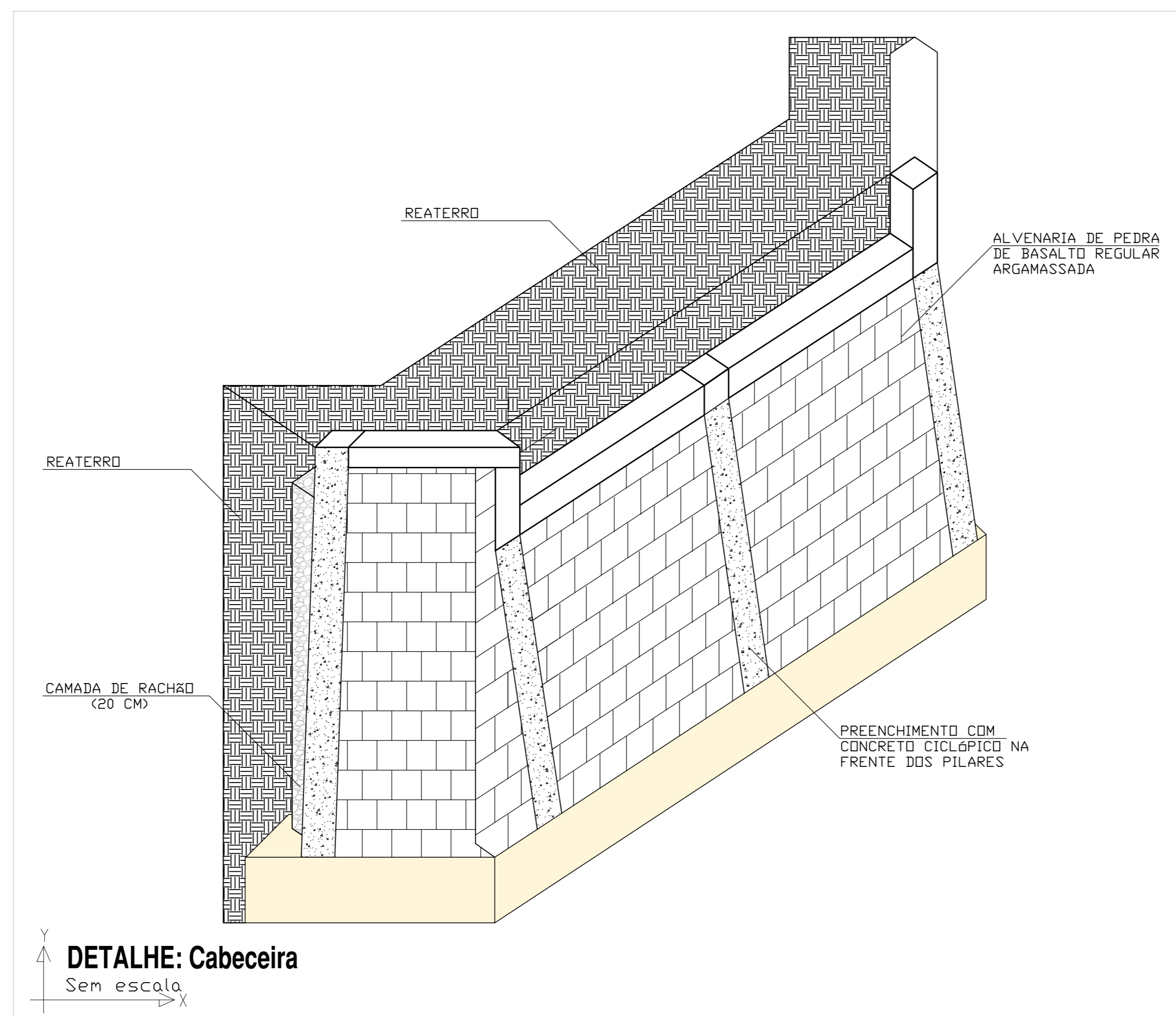
DETALHE: Cabeceira com Kit Transposição Sem escala
