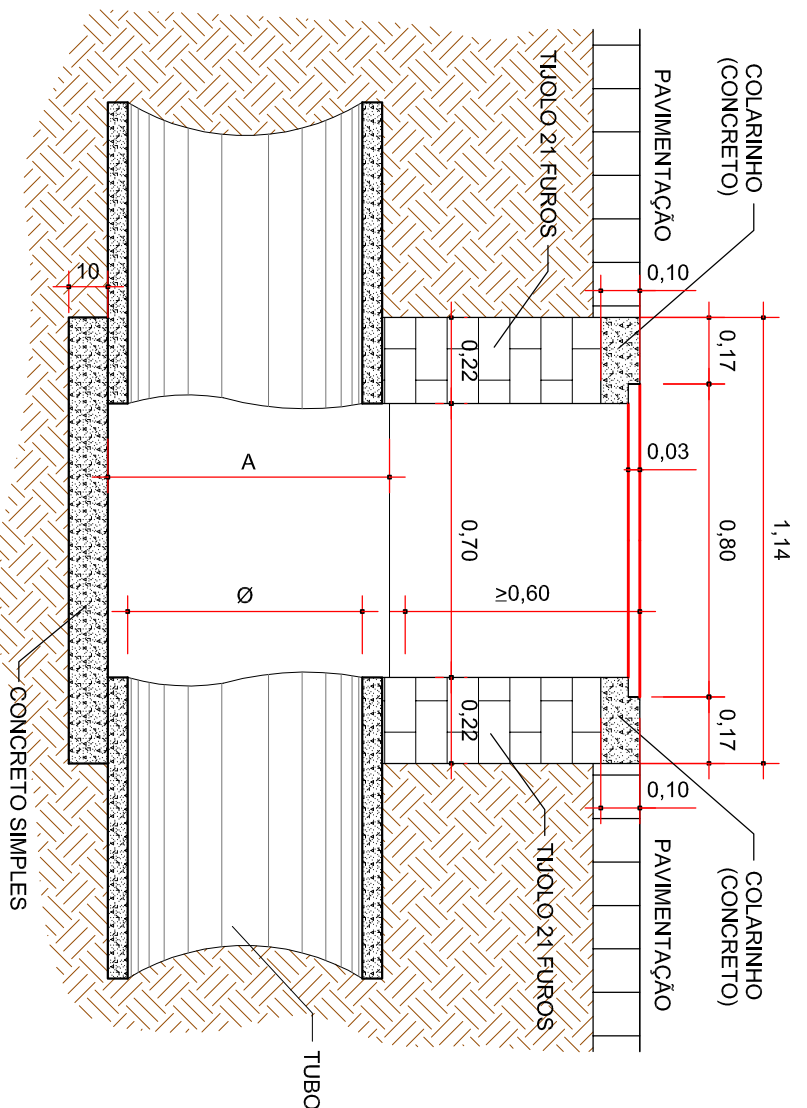
CORTE LONGITUDINAL (A A)
